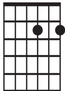
D6(add9)
